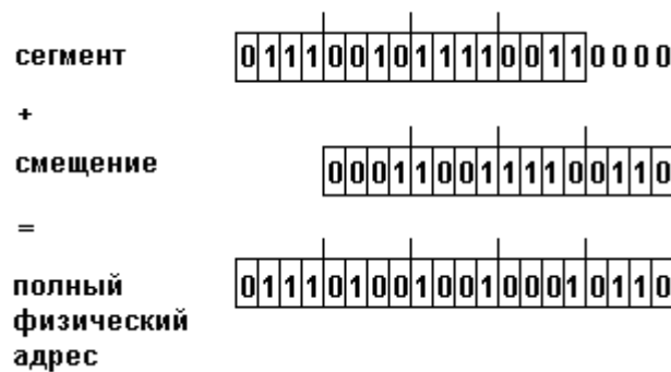
Рис 2.8. Вычисление полного адреса в микропроцессоре i8086.
