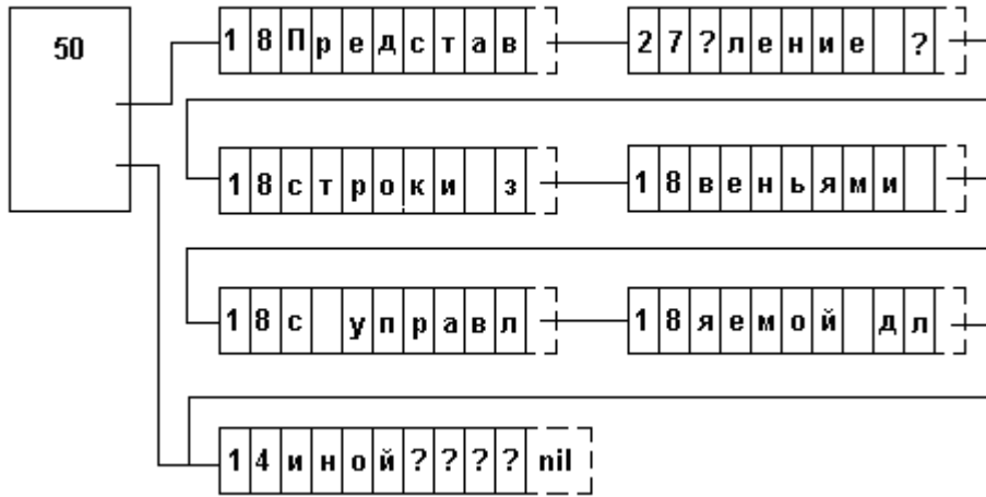
Рис.4.11. Представление строки звеньями управляемой длины
