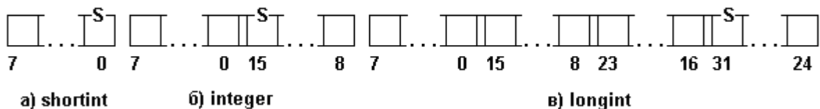
Рис. 2.3. Формат машинного представления чисел со знаком
