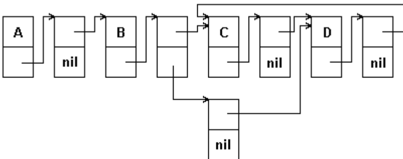
Рис.6.6. Машинное представление графа однотипными элементами
