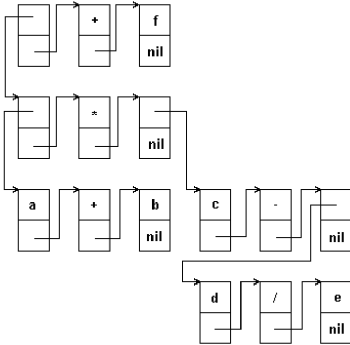
Рис.5.13. Схема списка, представляющего алгебраическое выражение
