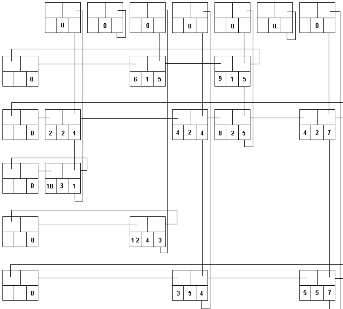
Рис. 3.7. Многосвязная структура для представления матрицы A
