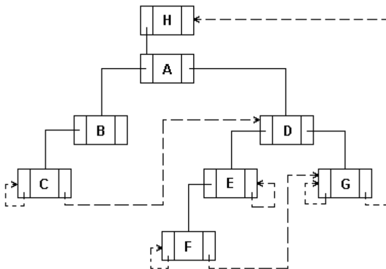
Рис. 6.28. Машинное связанное представление исходного дерева, представленного на рис.6.20 при нисходящем обходе с прошивкой
