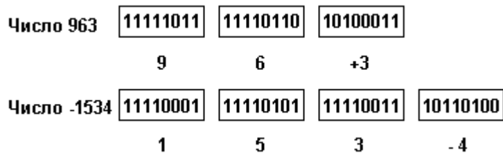
Рис.2.7. Машинное представление десятичных чисел в зонном формате
