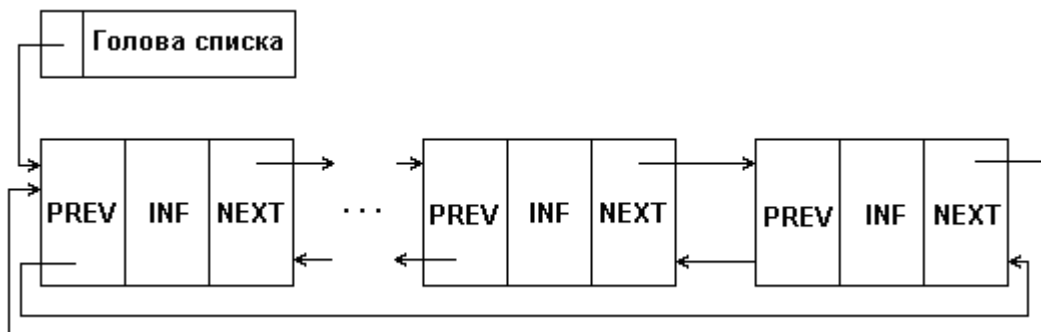
Рис.5.3. Структура кольцевого двухсвязного списка
