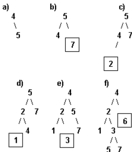
Рис. 6.35 Последовательное включение узлов в сбалансированное дерево.
