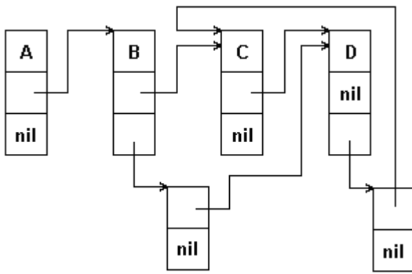
Рис.6.5. Машинное представление графа элементами двух типов
