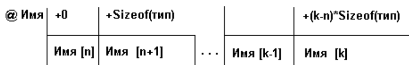
Рис. 3.1. Представление вектора в памяти
