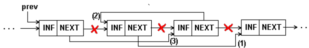
Рис.5.9. Перестановка соседних элементов 1-связного списка
