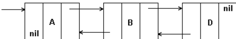
Рис.4.8. Представление строки двунаправленным связным списком
