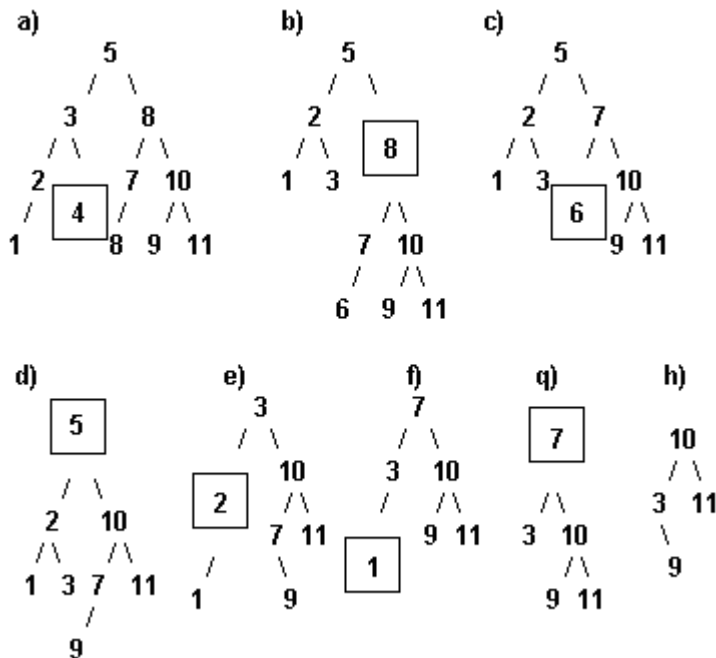
Рис.6.36 а..h Удаление узлов из сбалансированного дерева.
