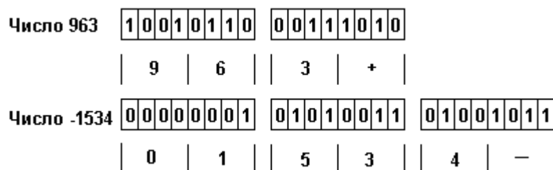
Рис.2.6. Машинное представление десятичных чисел в упакованном формате
