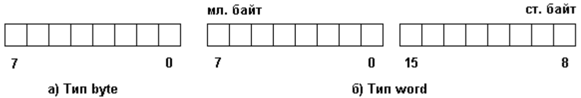
Рис. 2.2. Формат машинного представления беззнаковых чисел
