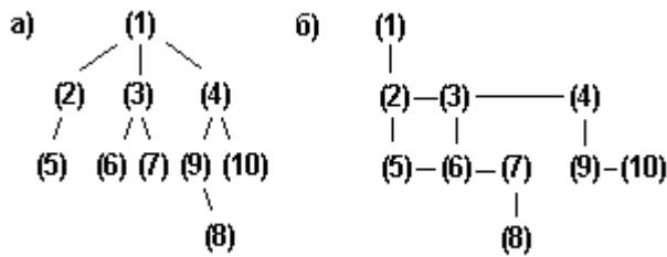
Рис. 6.22. Диаграммы дерева: а) исходное б) перестройка в бинарное
