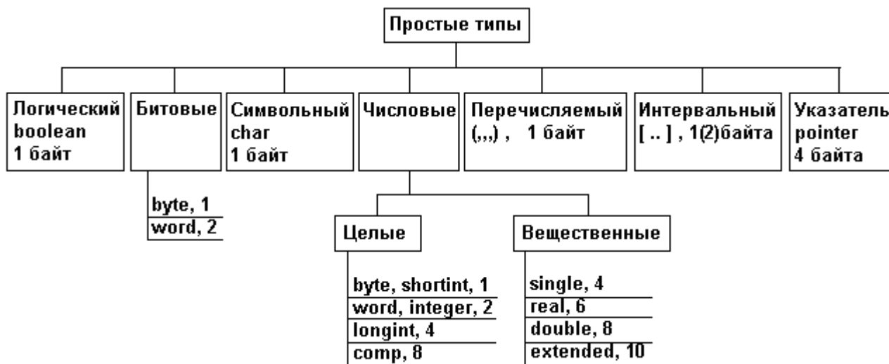
Рис. 2.1. Структура простых типов PASCAL.
