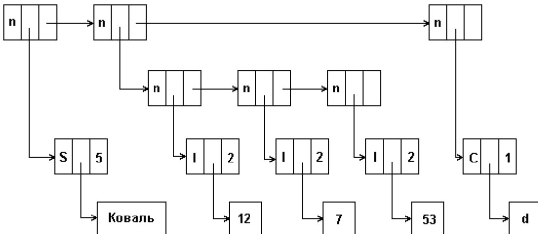
Рис.5.17. Пример представления списка элементами одного формата
