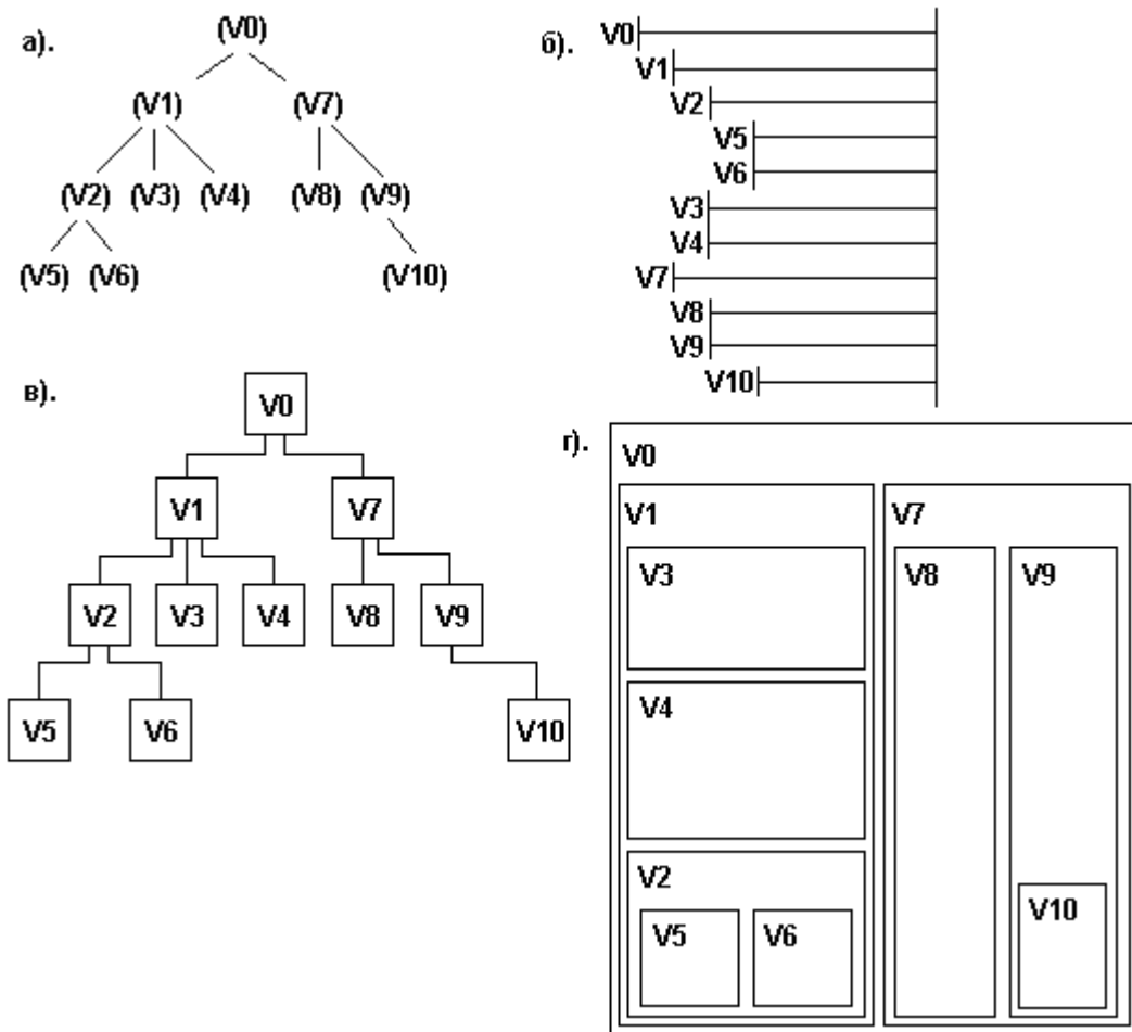
Рис.6.11. Представление дерева : а)- исходное дерево, б)- оглавление книг, в)- граф, г)- диаграмма Венна
