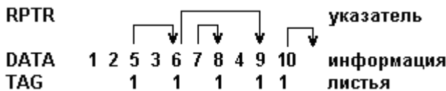
Рис. 6.23. Последовательное представление дерева методом опускания полей
