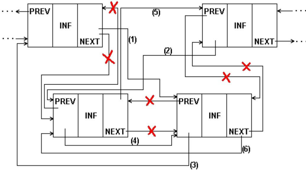
Рис.5.10. Перестановка соседних элементов 2-связного списка
