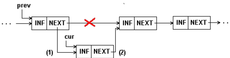
Рис.5.4. Вставка элемента в середину 1-связного списка
