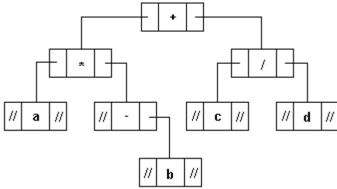
Рис. 6.32 Представление выражения в виде бинарного дерева.
