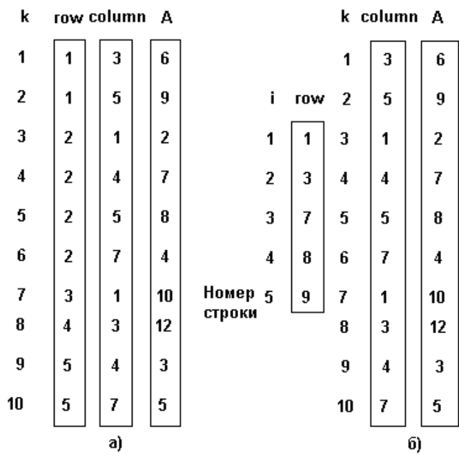
Рис. 3.5. Последовательное представление разреженных матриц.
