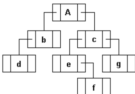
Рис. 6.21. Машинное связанное представление дерева представленного на рис.6.20
