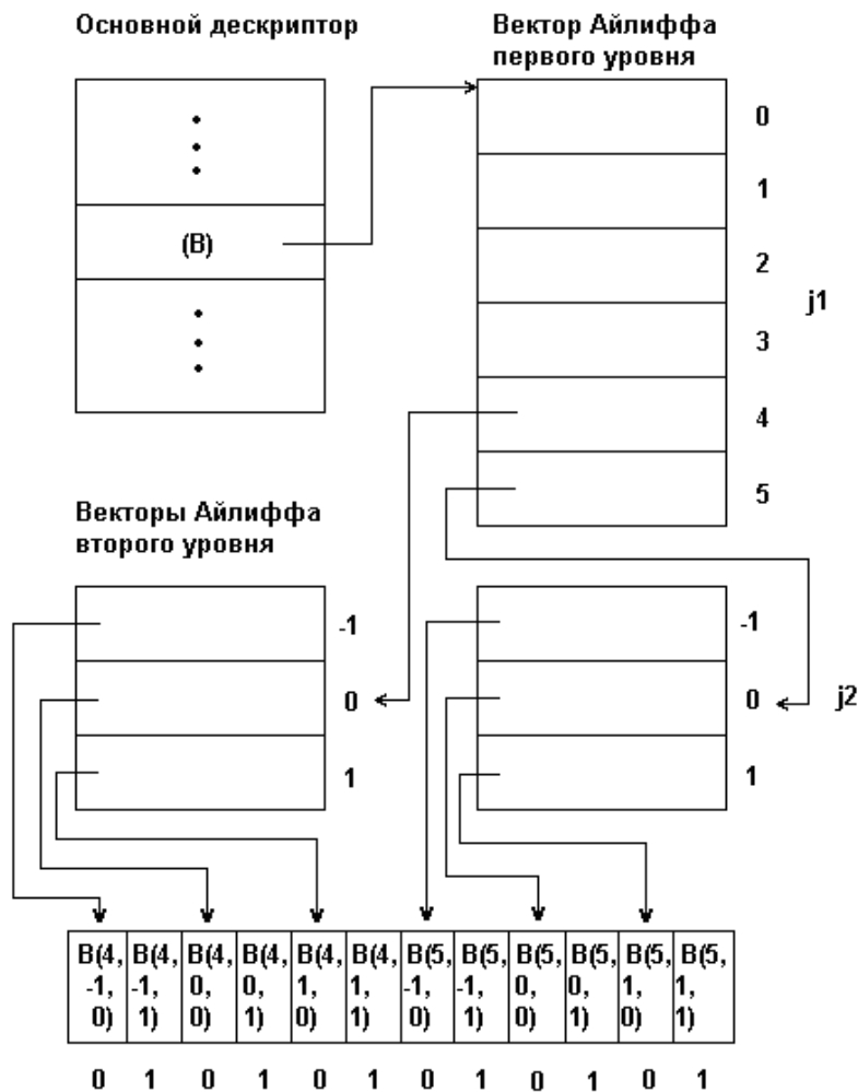
Рис. 3.4. Представление массивов с помощью векторов Айлиффа
