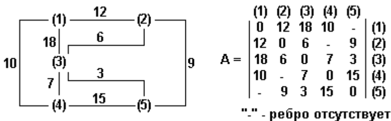
Рис.6.7. Часть дорожной карты, представленная в виде взвешенного графа и его матрицы смежности
