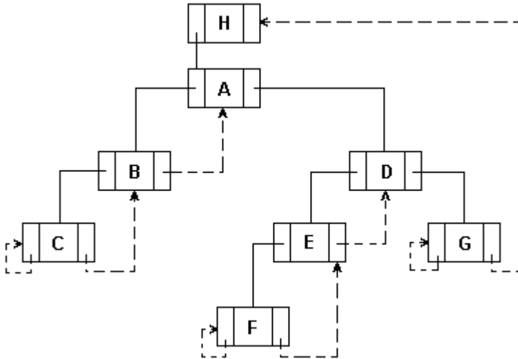
Рис. 6.29. Машинное связное представление дерева при смешанном обходе с прошивкой
